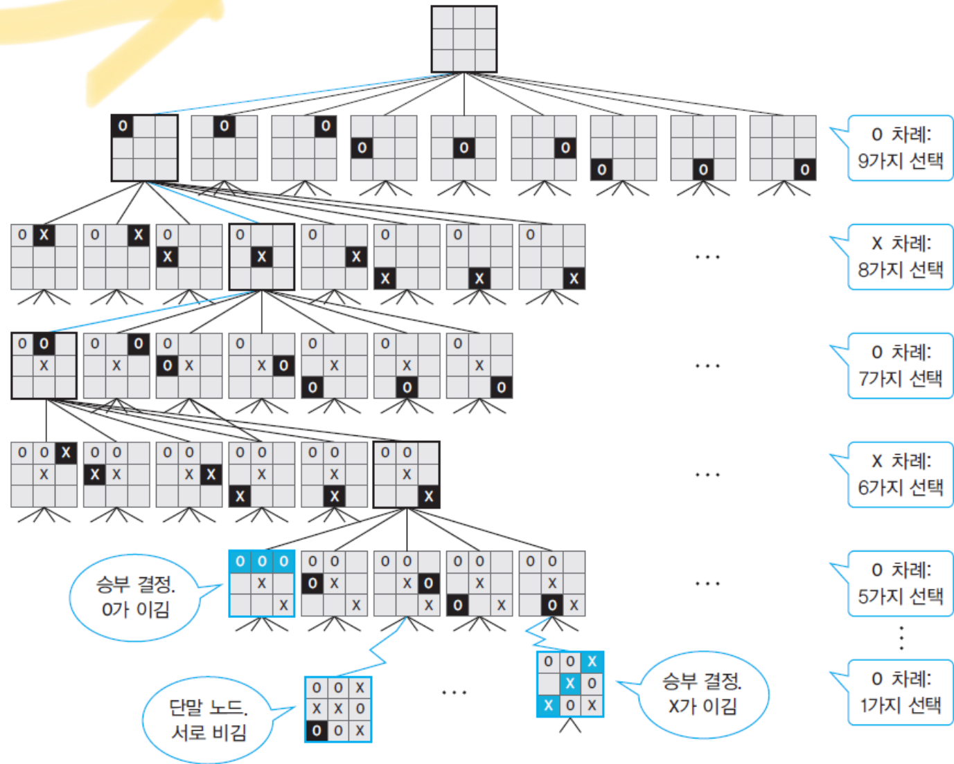
[그림 3.10] 틱택토 게임의 전체 상태공간트리
